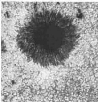
Figura 4. Mancha solar. Se observa la zona más oscura, umbra, rodeada de una zona
